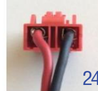
Posizione cablaggi su connettore / Cable positioning in the connector
